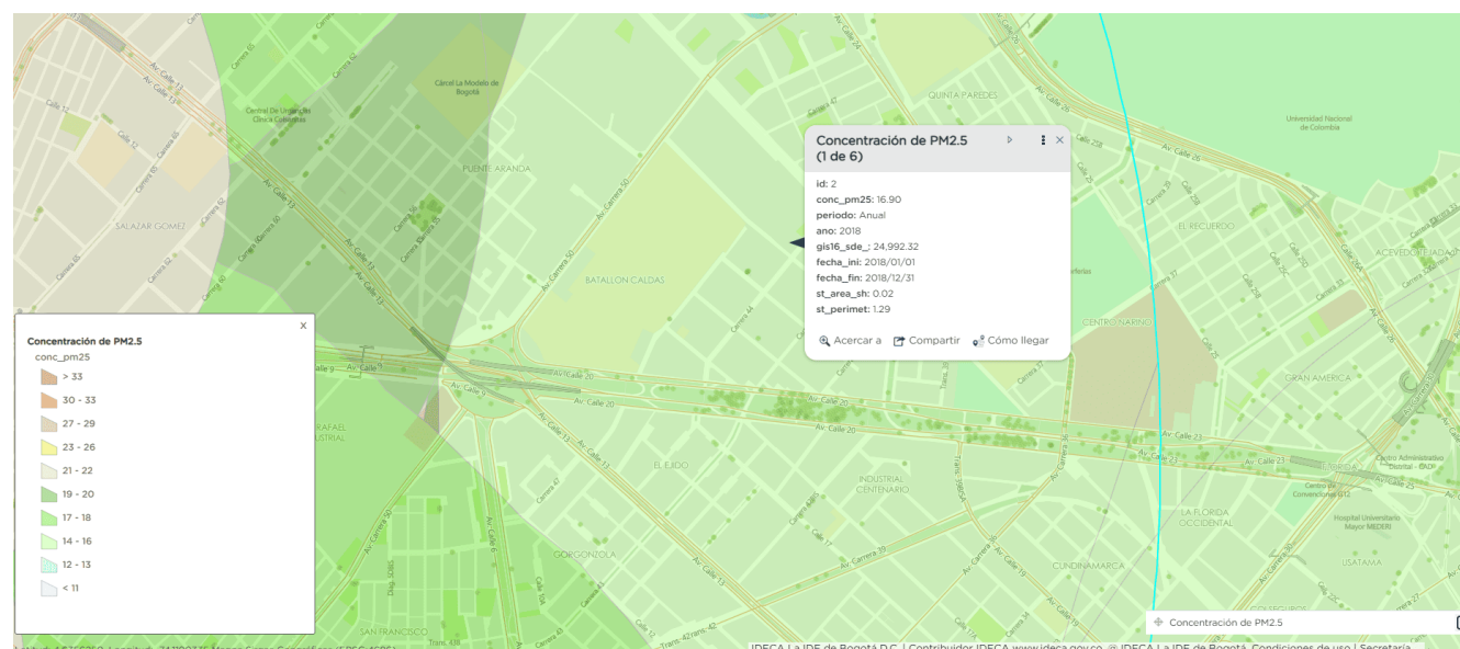
Ilustración 8. Concentración de material particulado PM2.5
